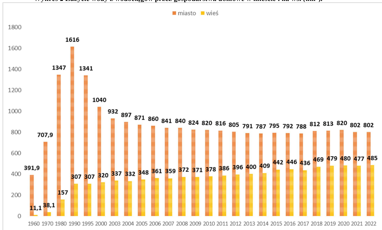
Wykres 2 Zużycie wody z wodociągów przez gospodarstwa domowe w mieście i na wsi (hm 3 ).
